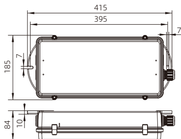
三防消防应急照明灯/标志灯
